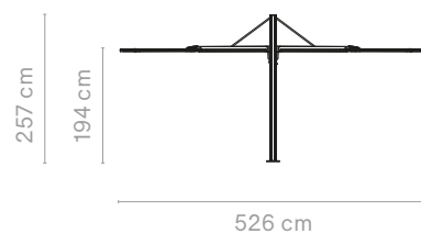
Sensu quattro diamond + grondverankering met paal verlengstuk
