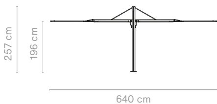
Sensu duo square + grondverankering met paal verlengstuk
