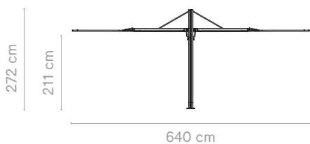
Sensu duo square + grondverankering met paal verlengstuk
